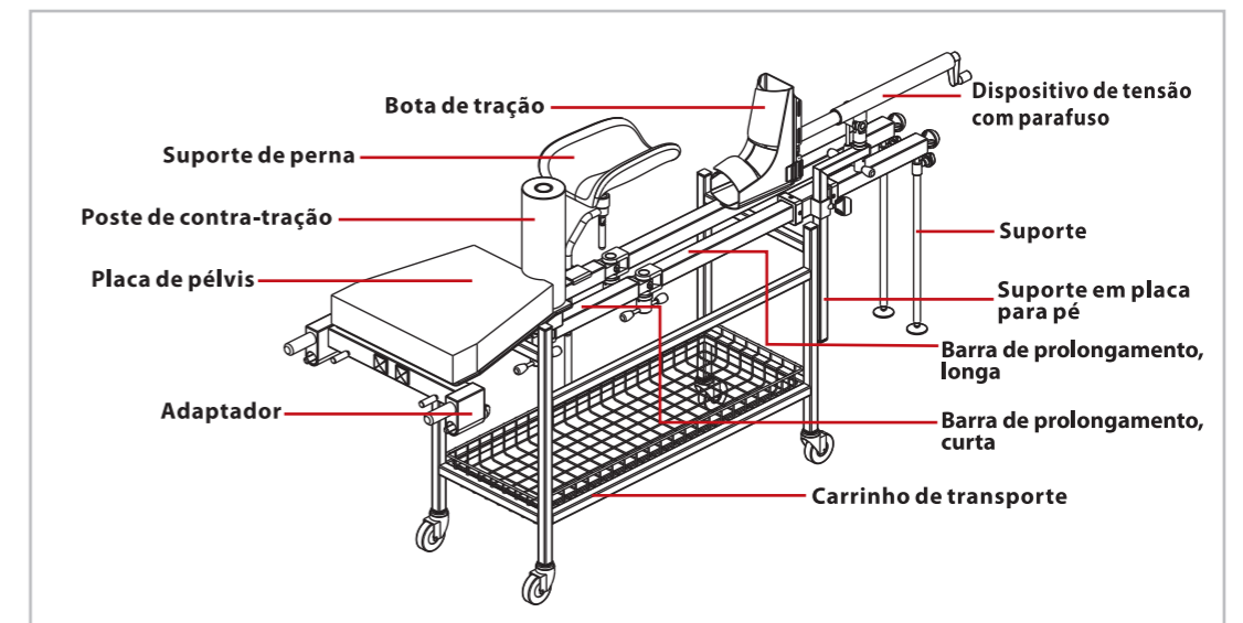
Extensão ortopédica 115-005691-00&115-005780-00 (Carrinho de transporte)
